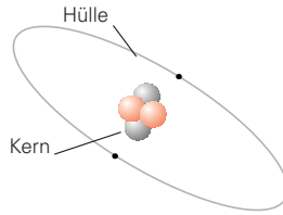
Helium-Atom Kern: 2 Protonen 2 Neutronen Hülle: 2 Elektronen
