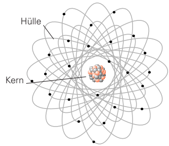
Uran-Atom 92 Protonen 146 Neutronen 92 Elektronen
